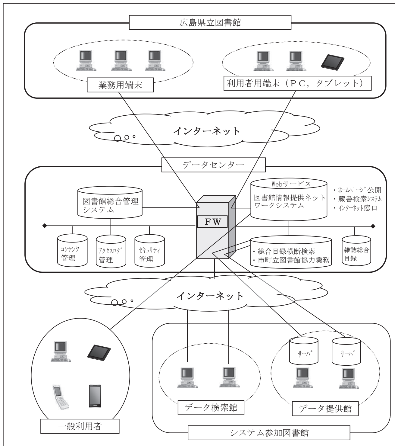
広島県立図書館情報提供システムネットワーク概要図
